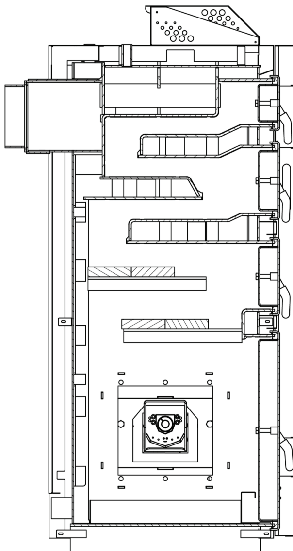
Rys. Rozmieszczenie płyt w kotle LE10 PELLET.
