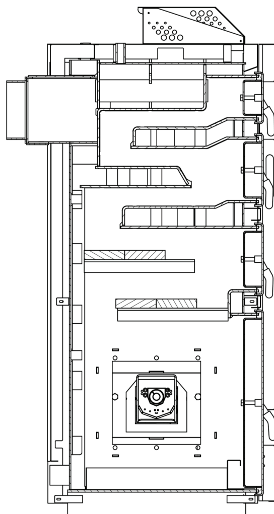
Rys. Poglądowy przekrój kotła LE10 PELLET w wersji NG
