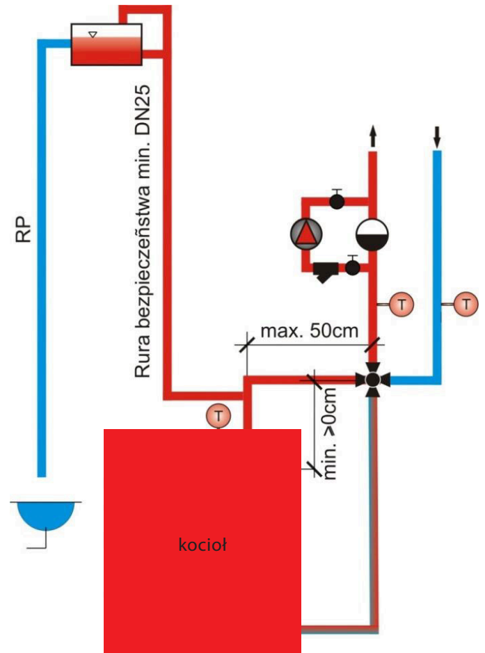
Rys. Schemat poglądowy umiejscowienia zaworu czterodrogowego.
