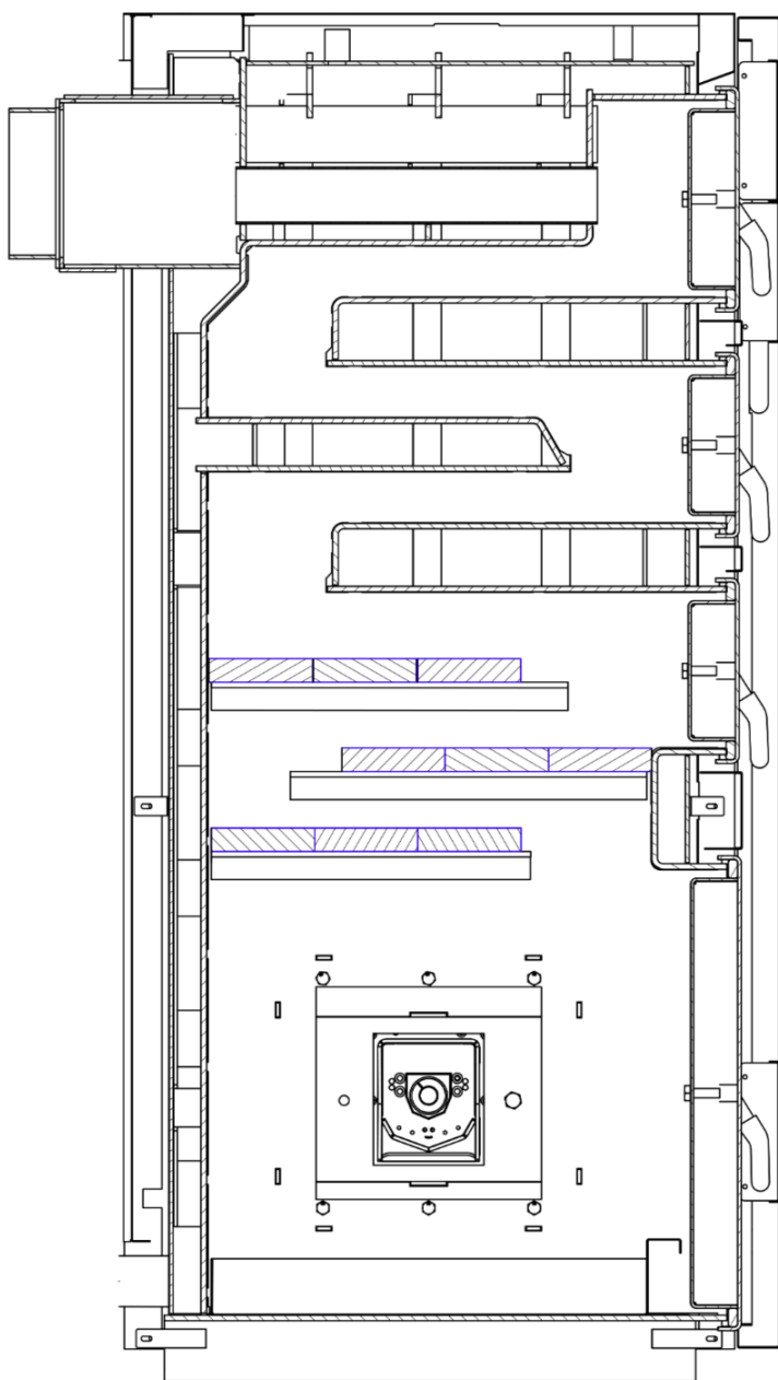
Rys. Rozmieszczenie płyt w kotle LE20 PELLET.
