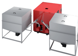
MAXI PELET 200 (zasobnik 3400l)
