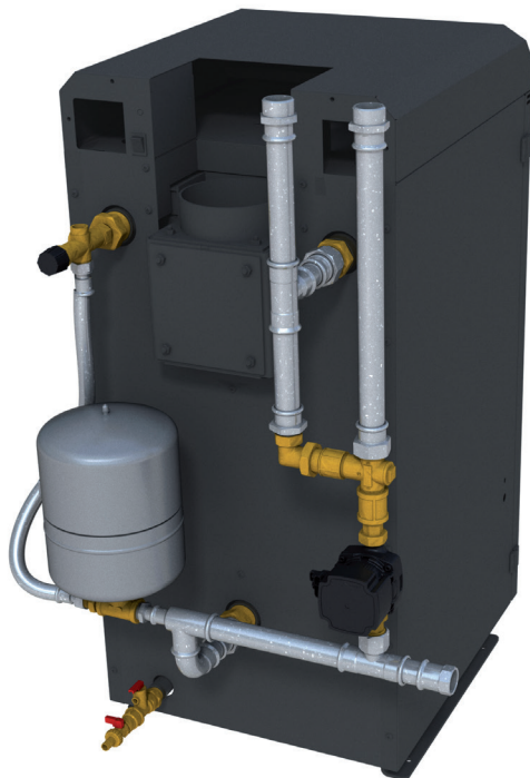
Przykład grupy bezpieczeństwa oraz grupy z zaworem termostaticznym dla kotła FRONTAL.
